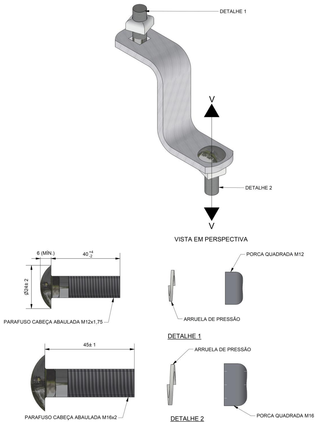
Figura 1 - Suporte Z
